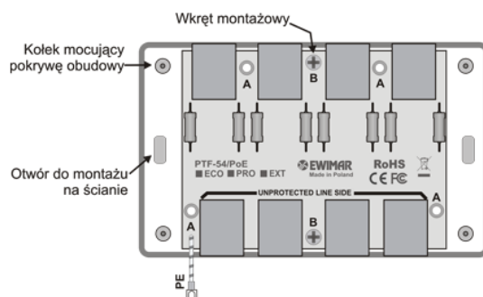
Sposób montażu modułu w obudowie
