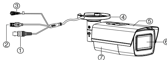
Kamera tubowa HD-TVI z obiektywem o zmiennej ogniskowej i funkcją motor-zoom (TVB-6103, TVB-6105, TVB-6106)
