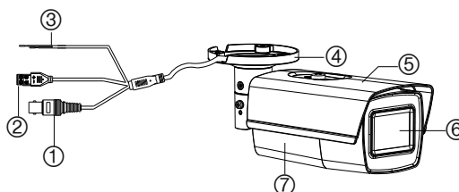
Rysunek 2: Kamera tubowa HD-TVI z obiektywem o zmiennej ogniskowej i funkcją motor-zoom (TVB-6101)
