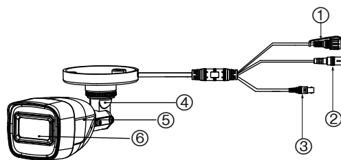
Rysunek 1: Kamera tubowa HD-TVI z obiektywem o stałej ogniskowej (TVB-6102, TVB-6104)
