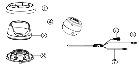
Rysunek 3: Kamera kopułowa typu turret HD-TVI z obiektywem o stałej ogniskowej do pracy przy słabym świetle (TVT-6103)
