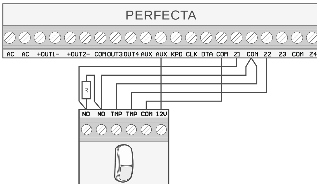
Rys. 15. Przykład podłączenia czujki NO w konfiguracji EOL.
