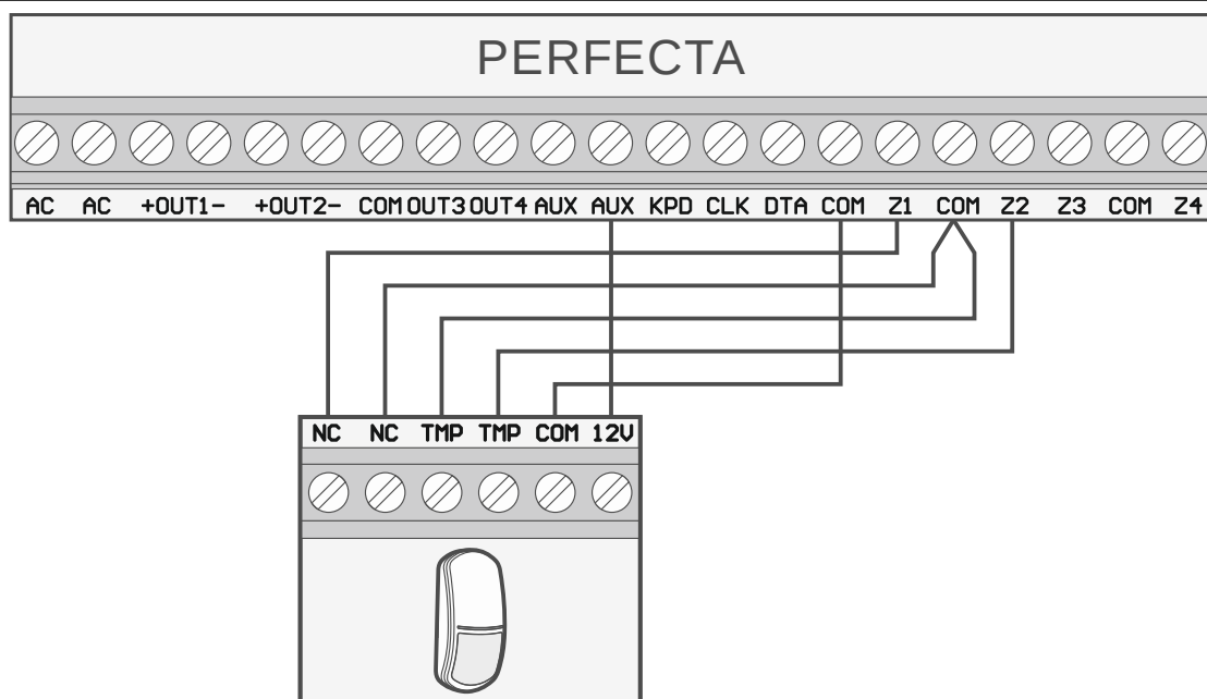
Rys. 13. Przykład podłączenia czujki NC (czujkę NO podłącz identycznie).
