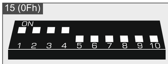
Rys. 10. Sposób ustawienia przełączników DIP-switch w ekspanderze INT-O.
