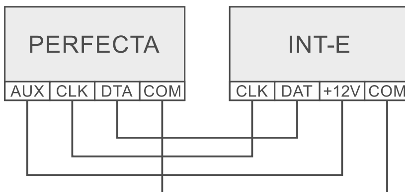
Rys. 7. Sposób podłączenia ekspandera INT-E do centrali.
