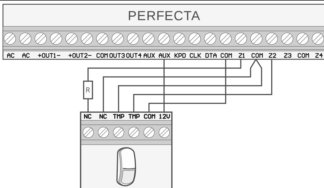
Rys. 14. Przykład podłączenia czujki NC w konfiguracji EOL.
