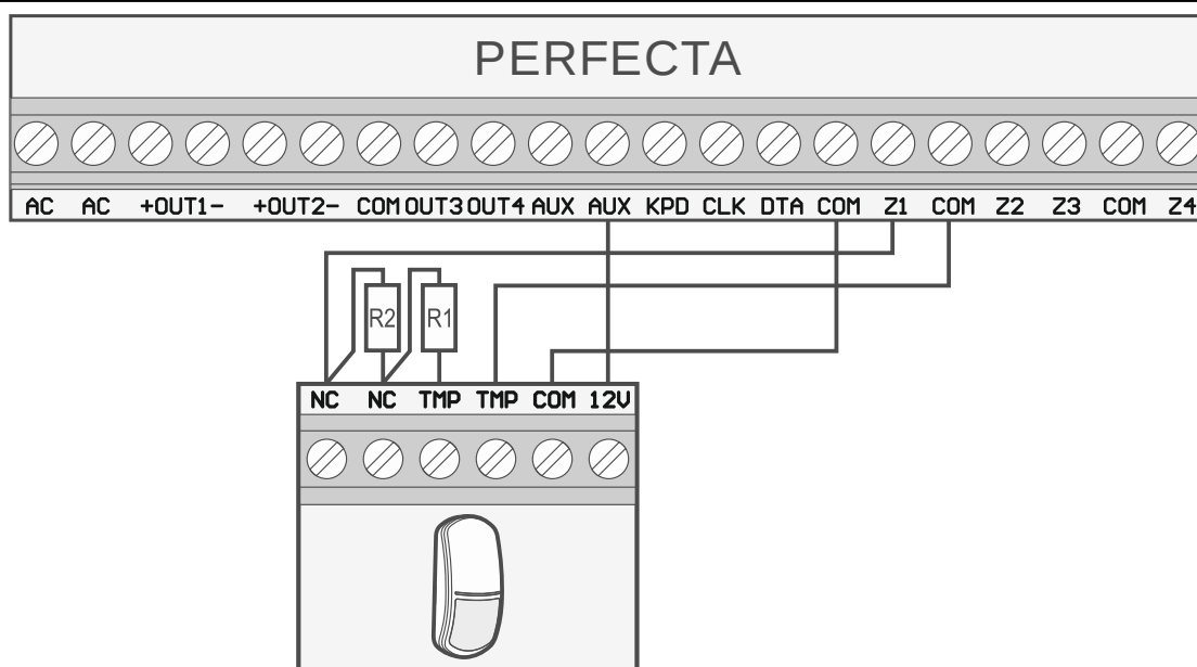
Rys. 16. Przykład podłączenia czujki NC w konfiguracji 2EOL (czujkę NO podłącz identycznie).
