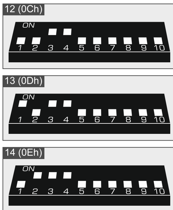
Rys. 8. Sposób ustawienia przełączników DIP-switch w ekspanderze INT-E.
