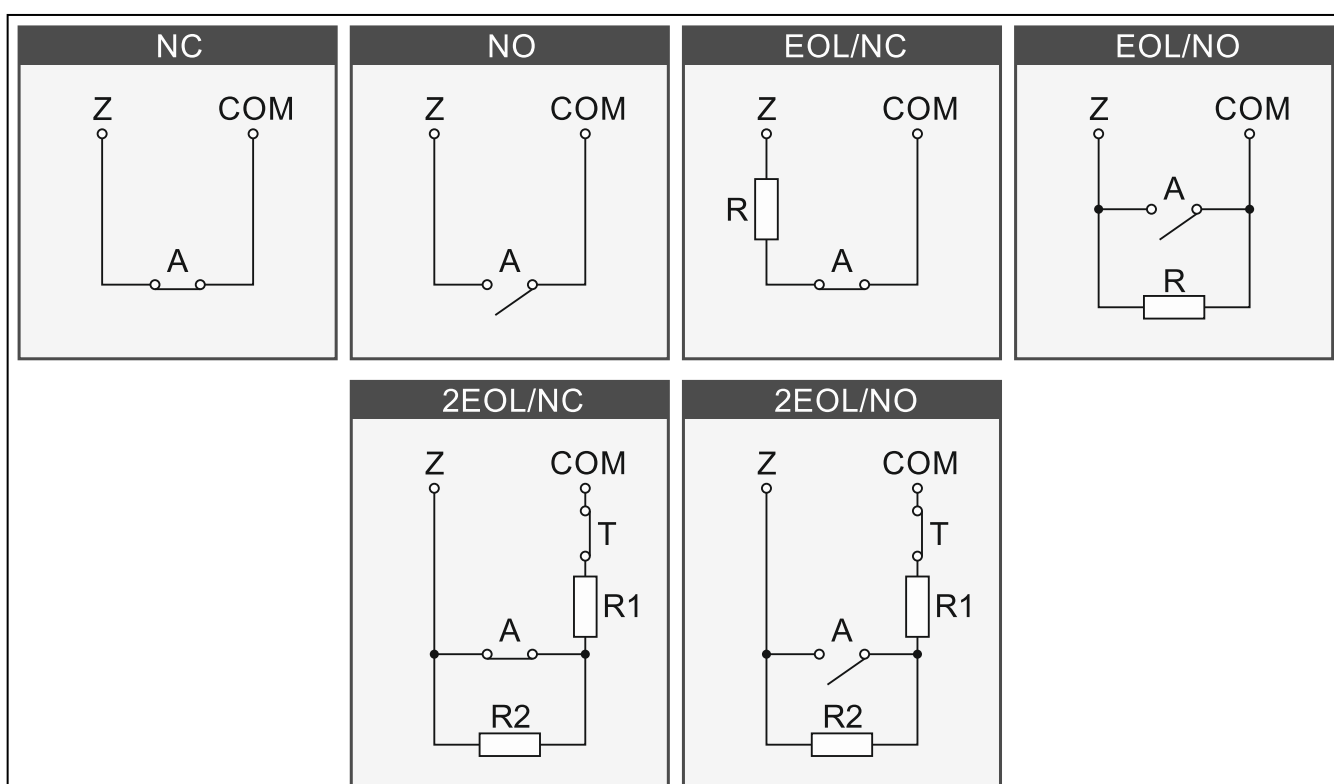
Rys. 12. Sposoby podłączania czujek do wejść. Wyjścia czujki oznaczone są literami: A - alarmowe, T – sabotażowe.
