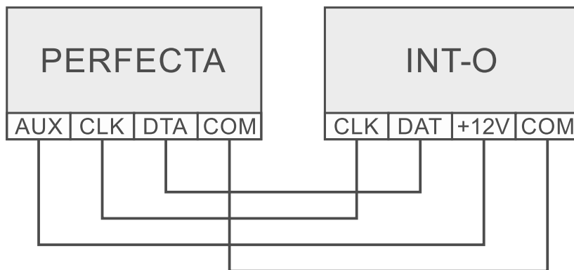
Rys. 9. Sposób podłączenia ekspandera INT-O do centrali.
