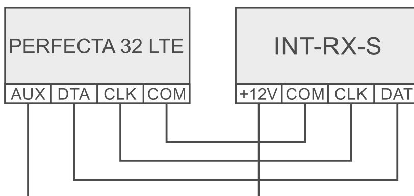
Rys. 5. Sposób podłączenia ekspandera INT-RX-S do centrali.
