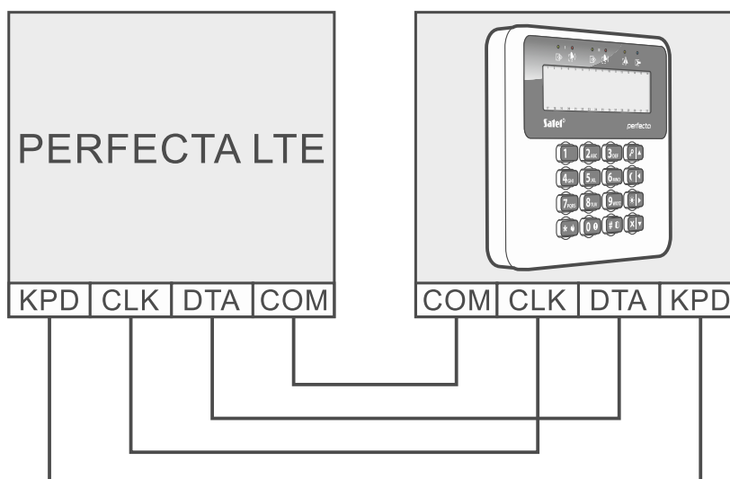
Rys. 4. Sposób podłączenia manipulatora do centrali.
