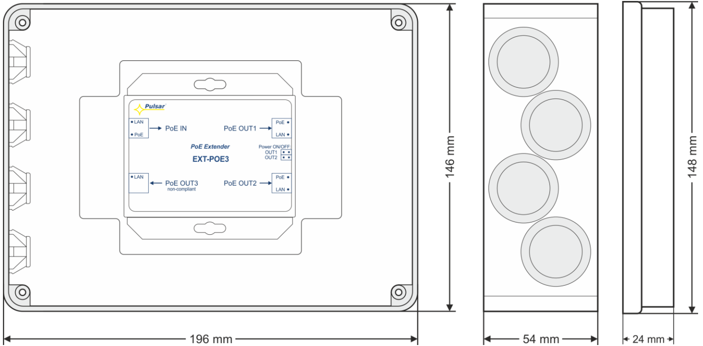
Rys. 1. Widok obudowy.
