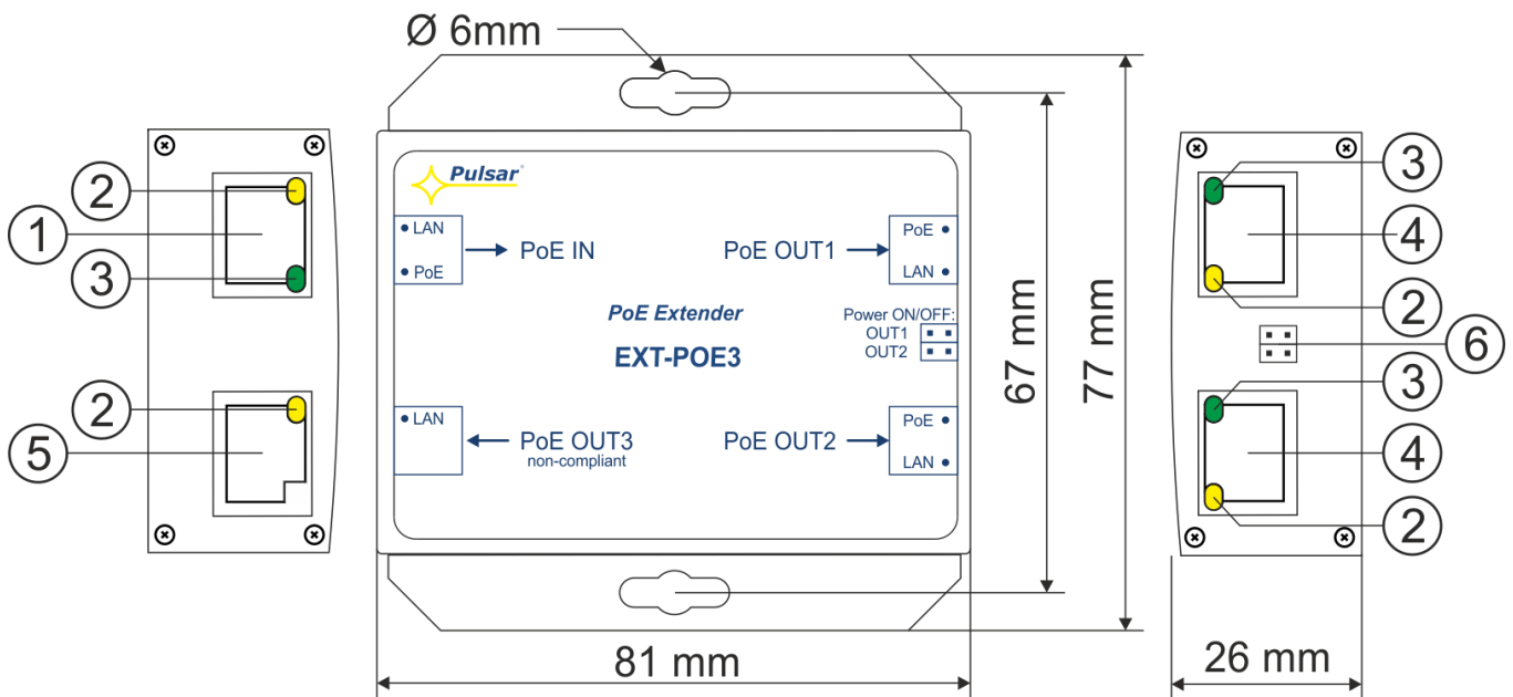
Rys. 2. Widok extender'a.
