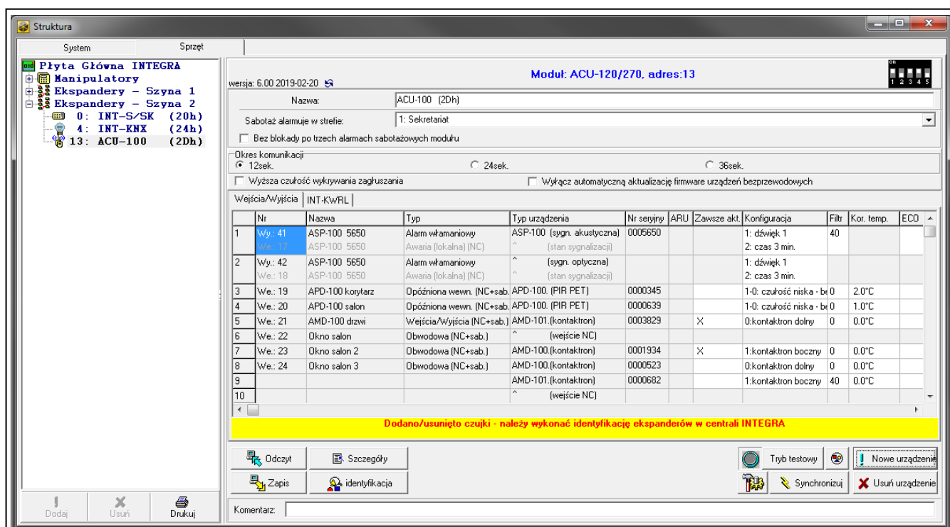
Rys. 20. Program DLOADX: informacje wyświetlane po zarejestrowaniu nowego urządzenia w kontrolerze połączonym do centrali INTEGRA / INTEGRA Plus.
