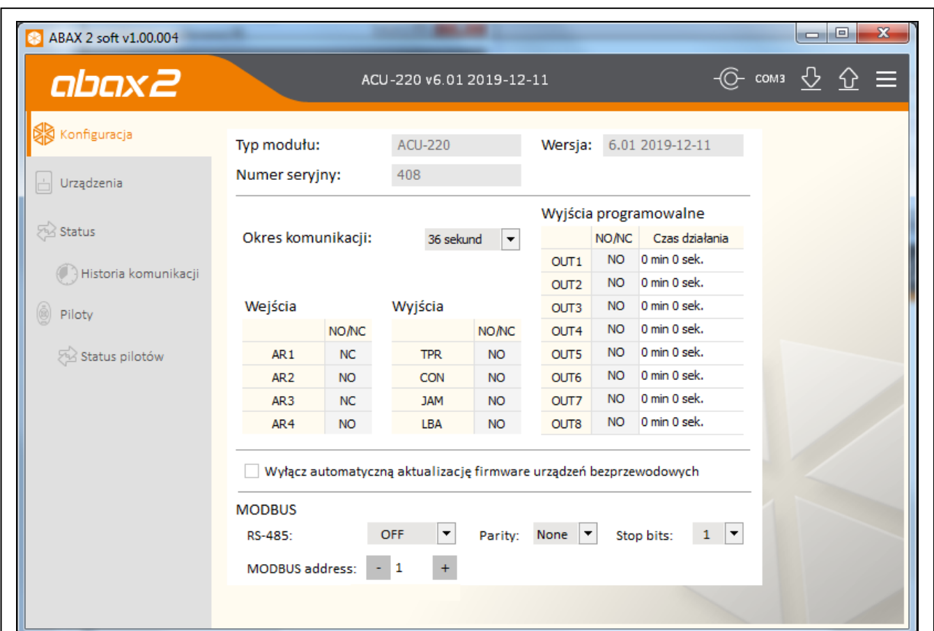
Rys. 11. Program ABAX 2 Soft: zakładka „Konfiguracja”.
