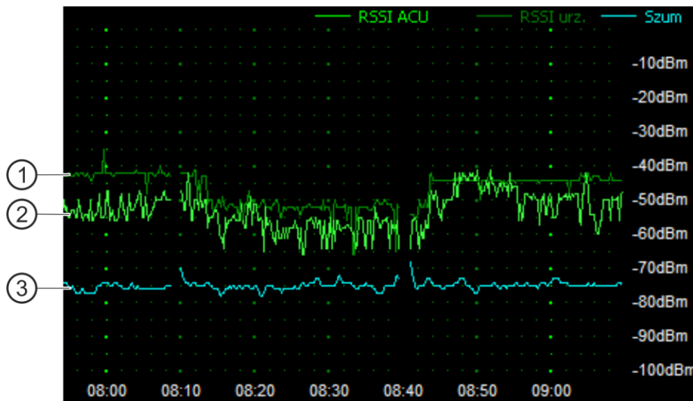
Rys. 16. Fragment wykresu przedstawiającego historię komunikacji.
