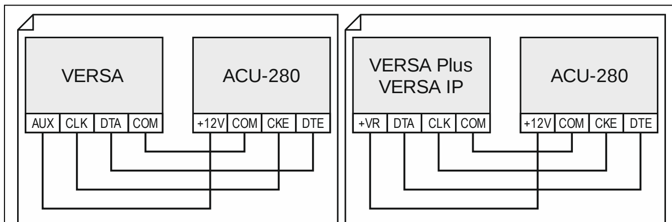
Rys. 7. Sposób podłączenia kontrolera do centrali VERSA / VERSA Plus / VERSA IP.
