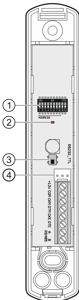
Rys. 1. Płytki elektroniki kontrolera.
