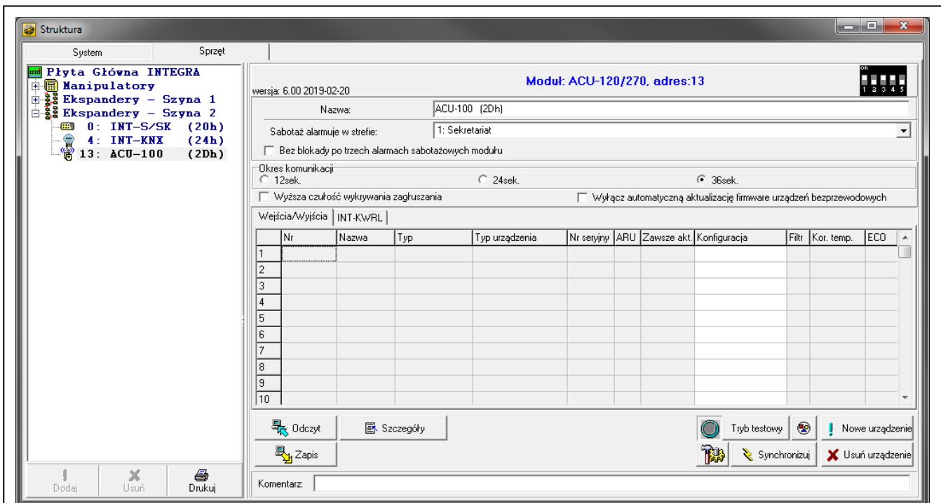
Rys. 21. Program DLOADX: parametry i opcje kontrolera podłączonego do centrali INTEGRA / INTEGRA Plus.
