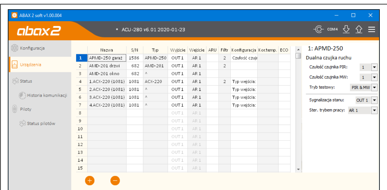
Rys. 12. Program ABAX 2 Soft: zakładka „Urządzenia”.
