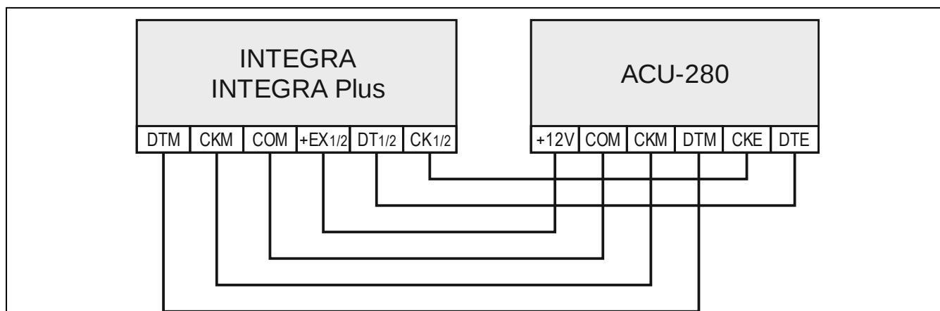
Rys. 6. Sposób podłączenia kontrolera do centrali INTEGRA / INTEGRA Plus.
