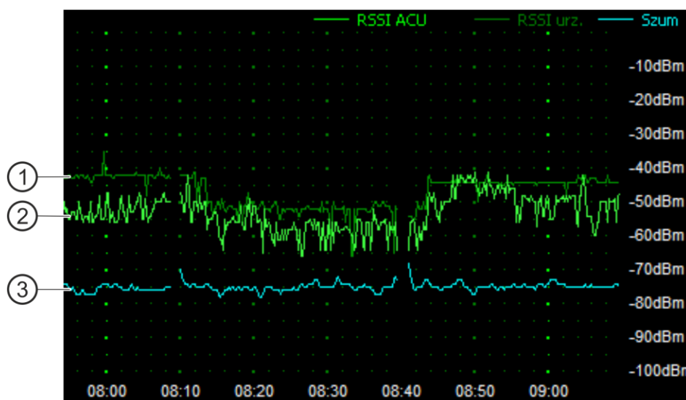
Rys. 16. Fragment wykresu przedstawiającego historię komunikacji.
