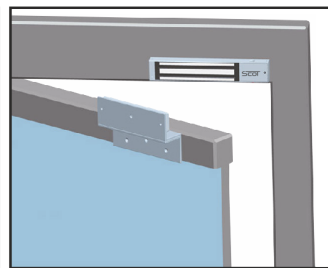
Montaż z uchwytem BK-600ZL2, BK-600ZLC2
