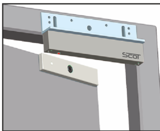
Montaż z uchwytem BK-600L2, BK-600LC2
