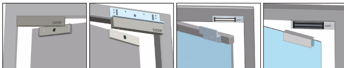
Montaż standardowy / z uchwytem BK-600L
