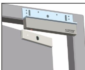
Montaż z uchwytem BK-800L, BK-800LC
