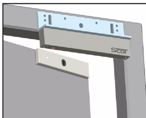
Montaż z uchwytem BK-800L2, BK-800LC2
