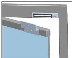
Montaż z uchwytem BK-800ZL2
