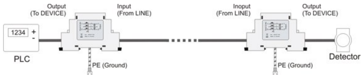
Schemat prawidłowego zabezpieczenia obwodu wejścia / wyjścia
